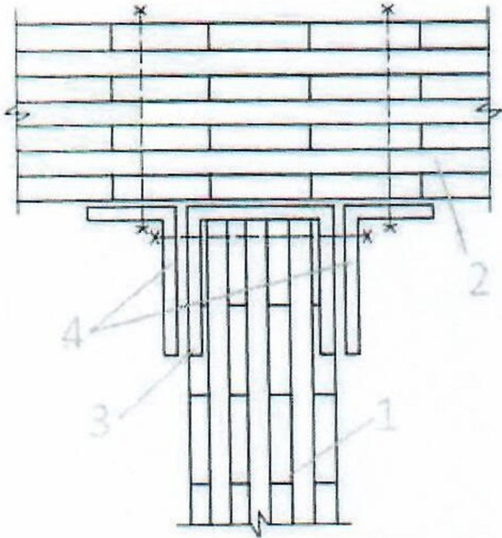
▲ Obr. 7 Náčrt spoje membrány 1 a obvodové stěny 2. Membrána je opatřena přilepeným kovovým profilem 3 a propojena se stěnou úhelníky 4 a šrouby.
