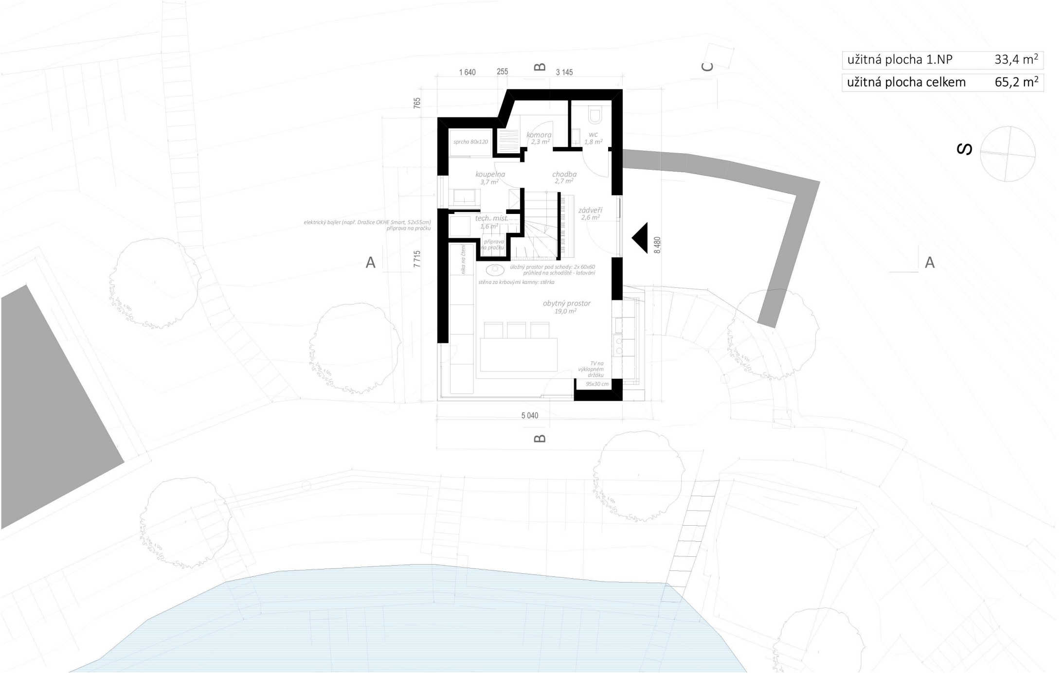
PŮDORYS 1. NP
