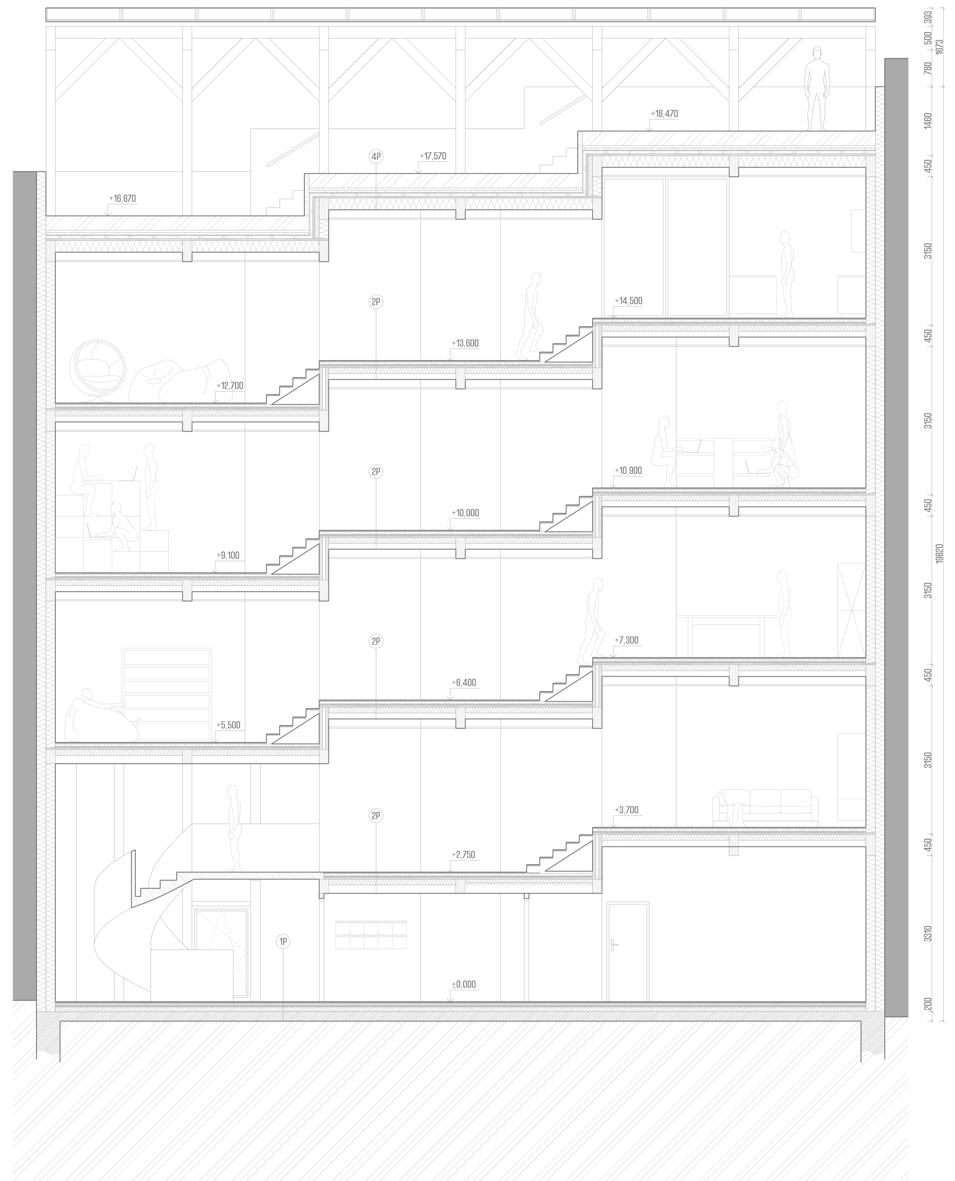
JIŽNÍ ŘEZ
