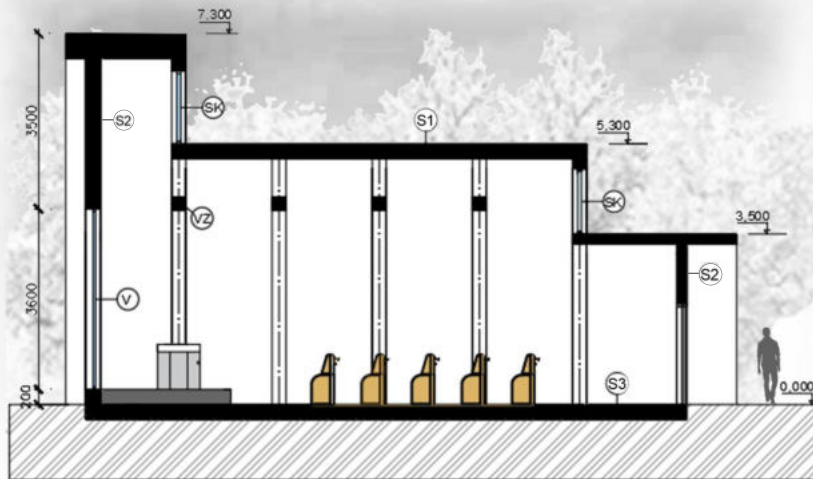
ŘEZ B-B'
