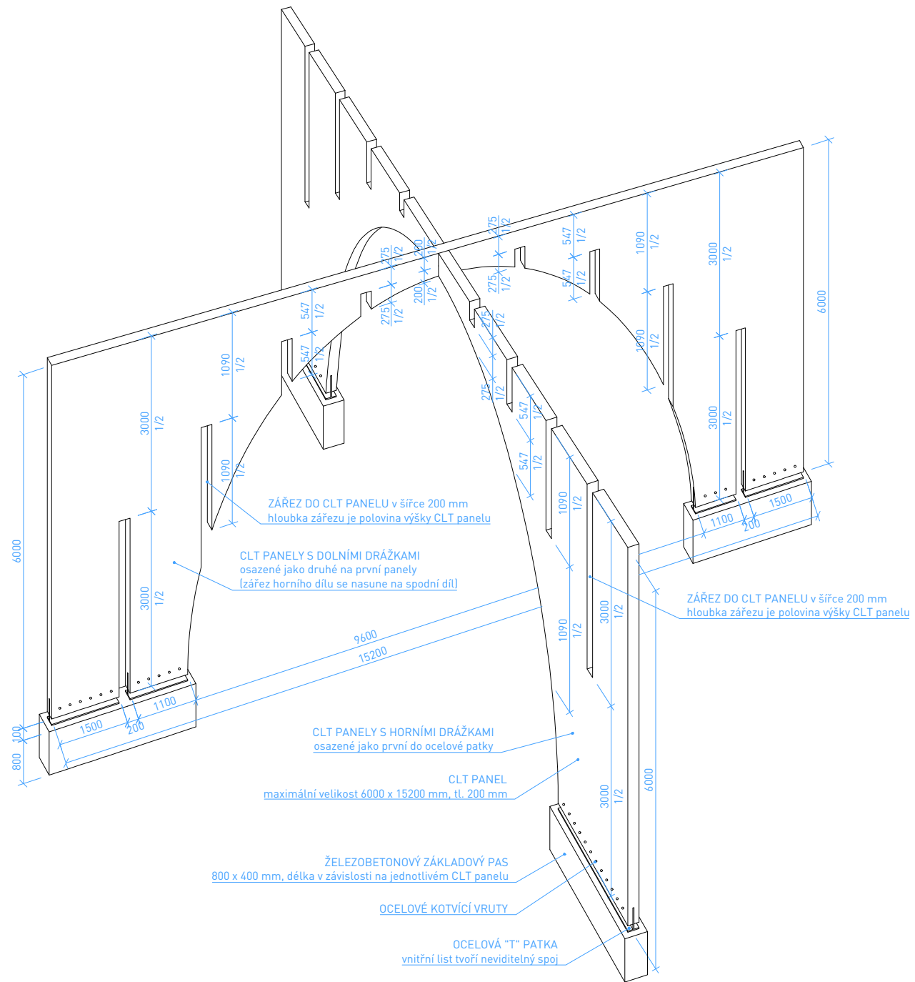
AXONOMETRIE OSAZENÍ CLT PANELŮ
