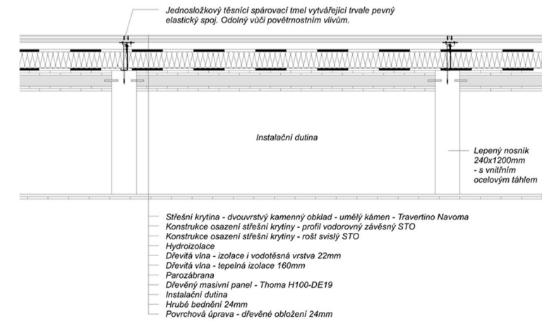
A Skladba hlavní nosné konstrukce včetně obvodového pláště
