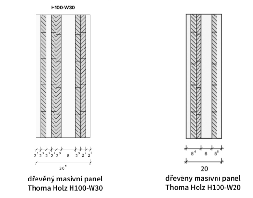
B Skladba vnitřních nosných stěn C Skladba vnitřních stěn
