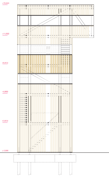
východní pohled m 1:100
