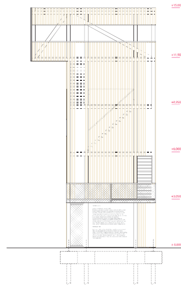
západní pohled m 1:100
