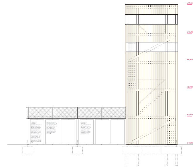
jižní pohled m 1:100
