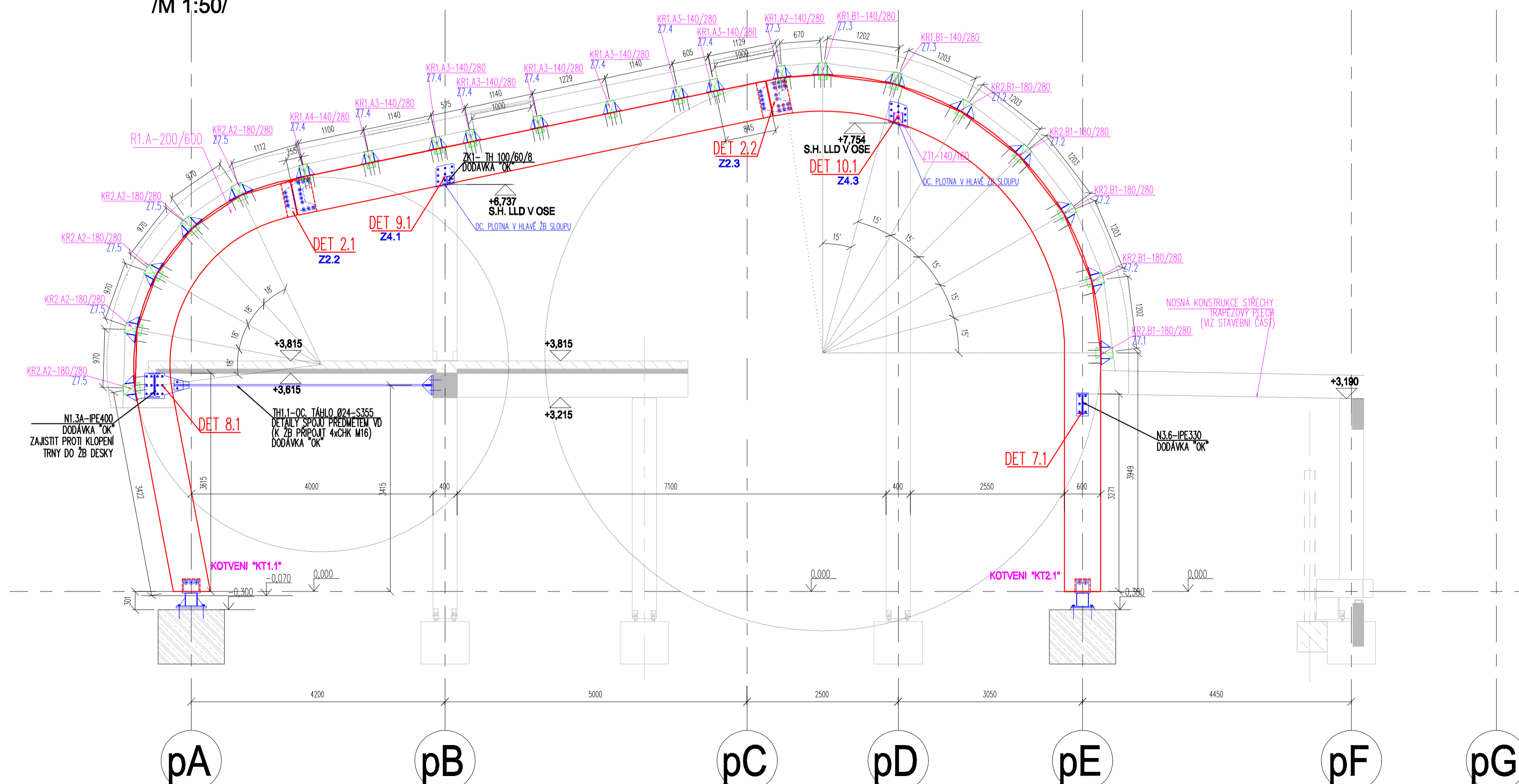
ŘEZ S.21 - OSA "p2" /M 1:50/
