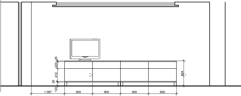
POHLED 1
