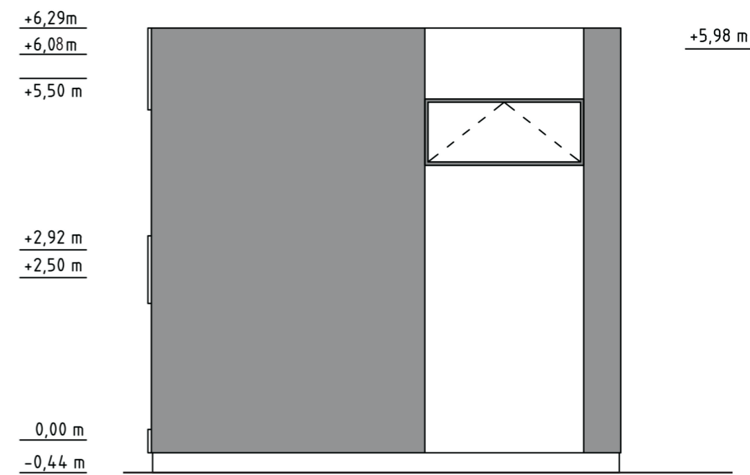
východní pohled
