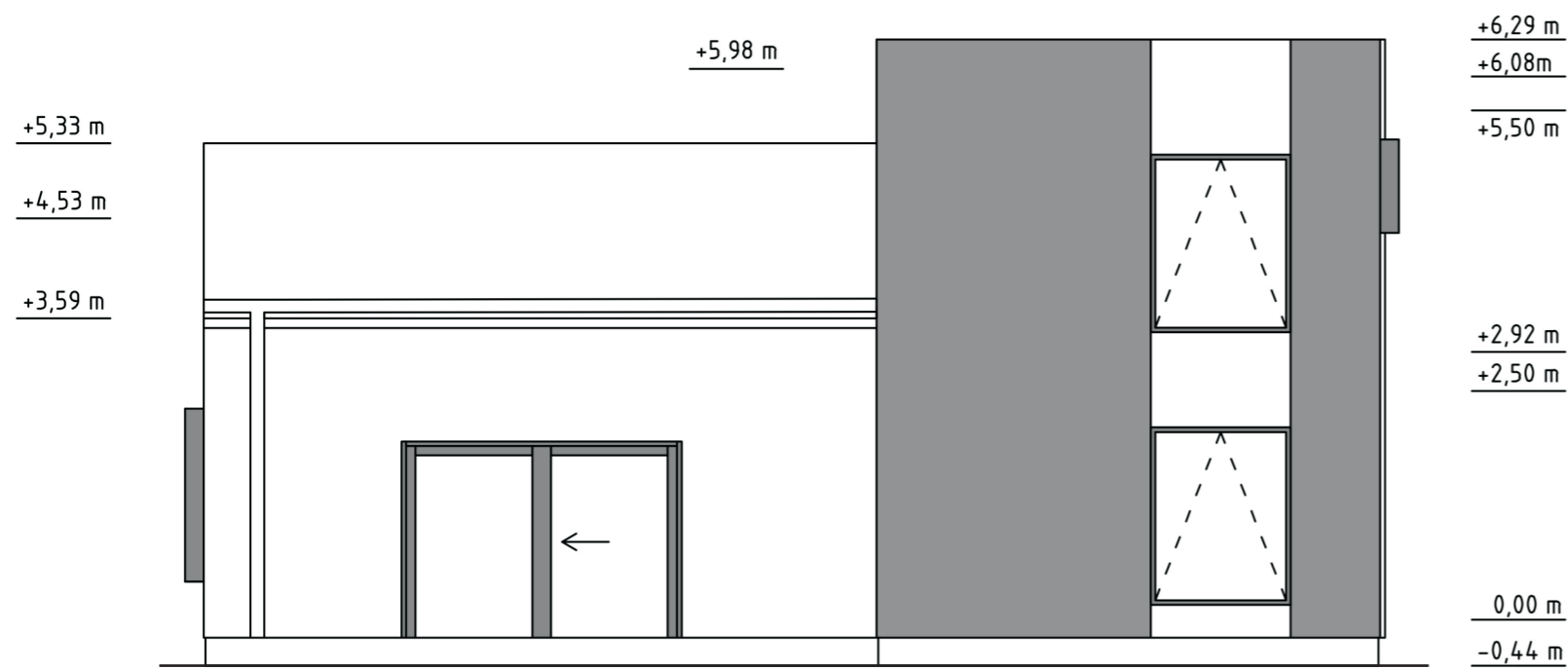
jižní pohled
