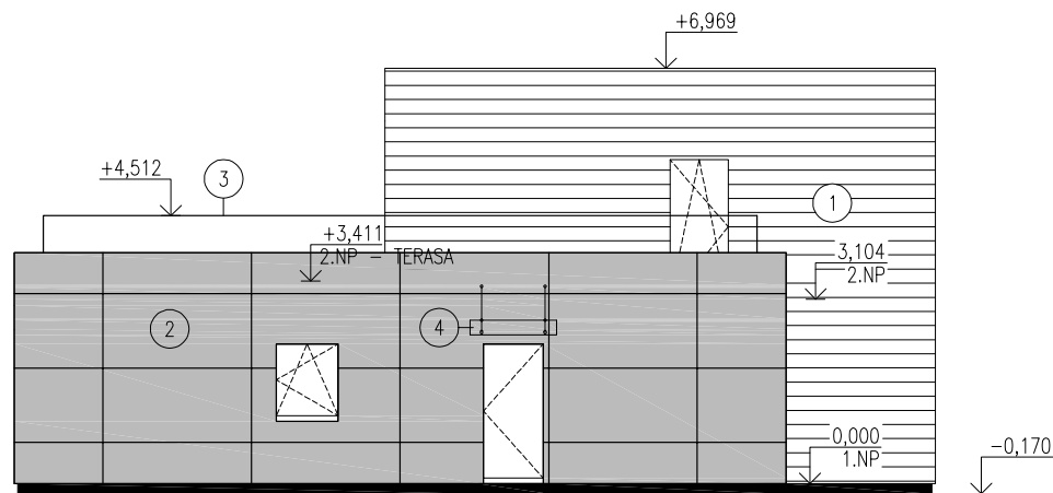
SEVEROVÝCHODNÍ POHLED
