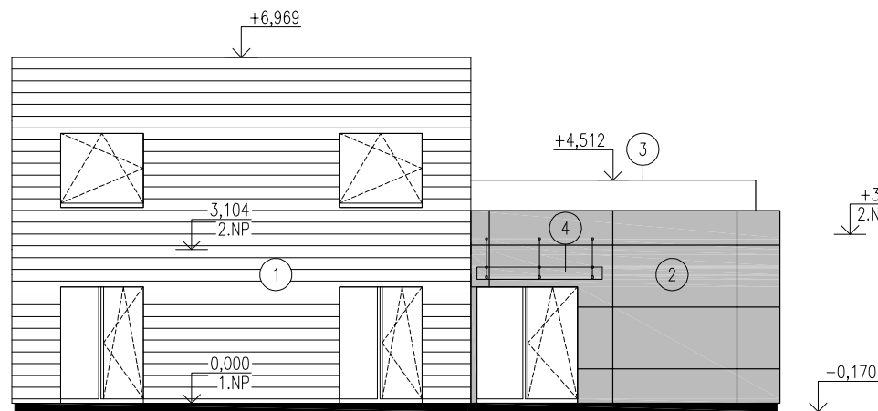
JIHOZÁPADNÍ POHLED
