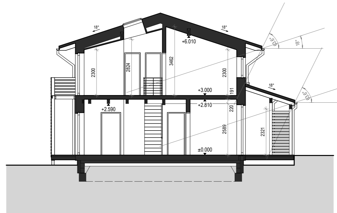
ŘEZ C-C'
