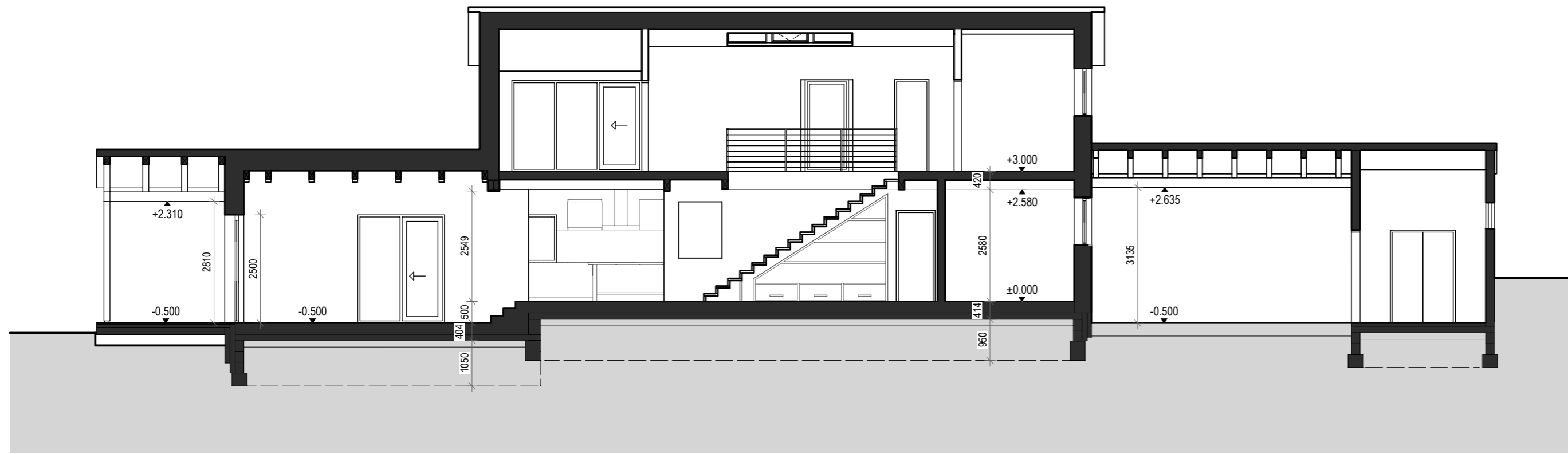
ŘEZ A-A'
