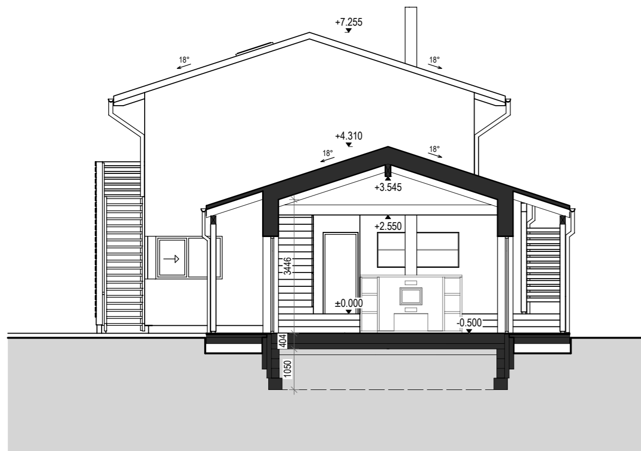
ŘEZ B-B'
