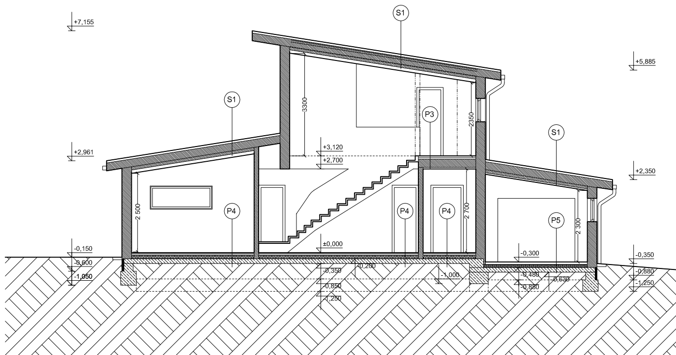
ŘEZ B-B
