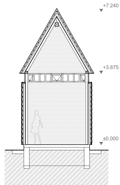
ŘEZ PŘÍČNÝ
