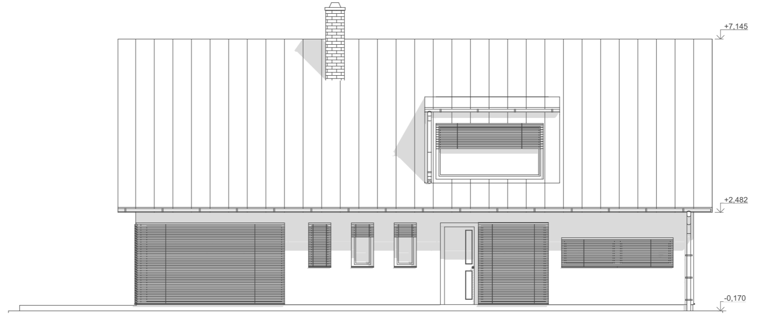
Pohled: východní
