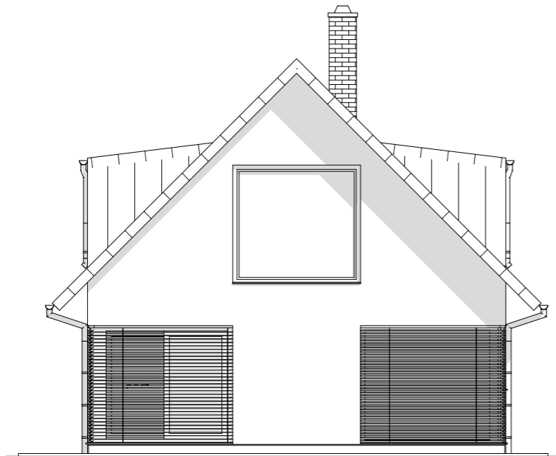
Pohled: jižní
