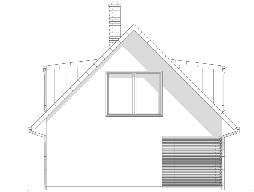
Pohled: severní
