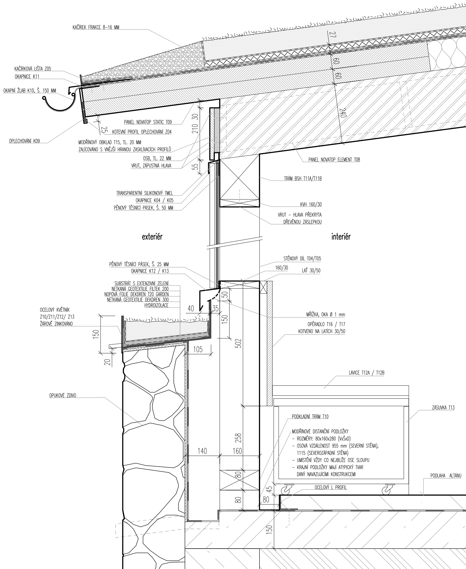
detail parapetu a střechy
