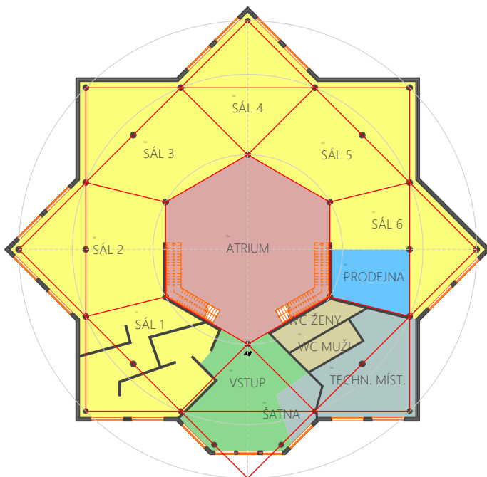
PŮDORYS 1. NP
