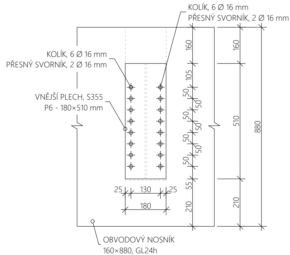
DETAIL C3 ŘEZ B-B
