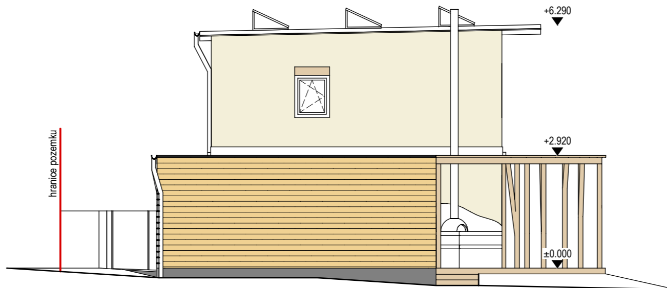
POHLED ZÁPADNÍ
