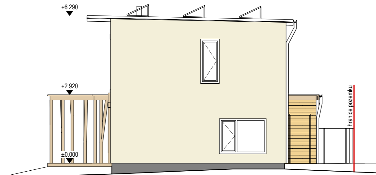
POHLED VÝCHODNÍ
