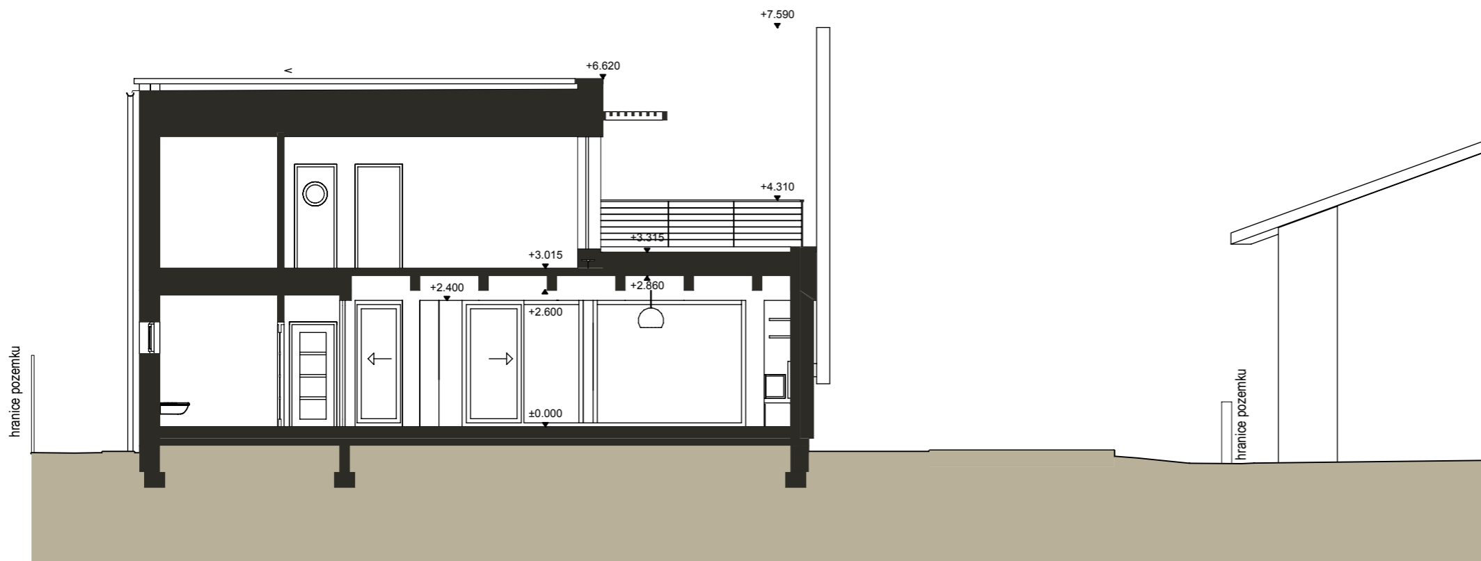
ŘEZ A-A'
