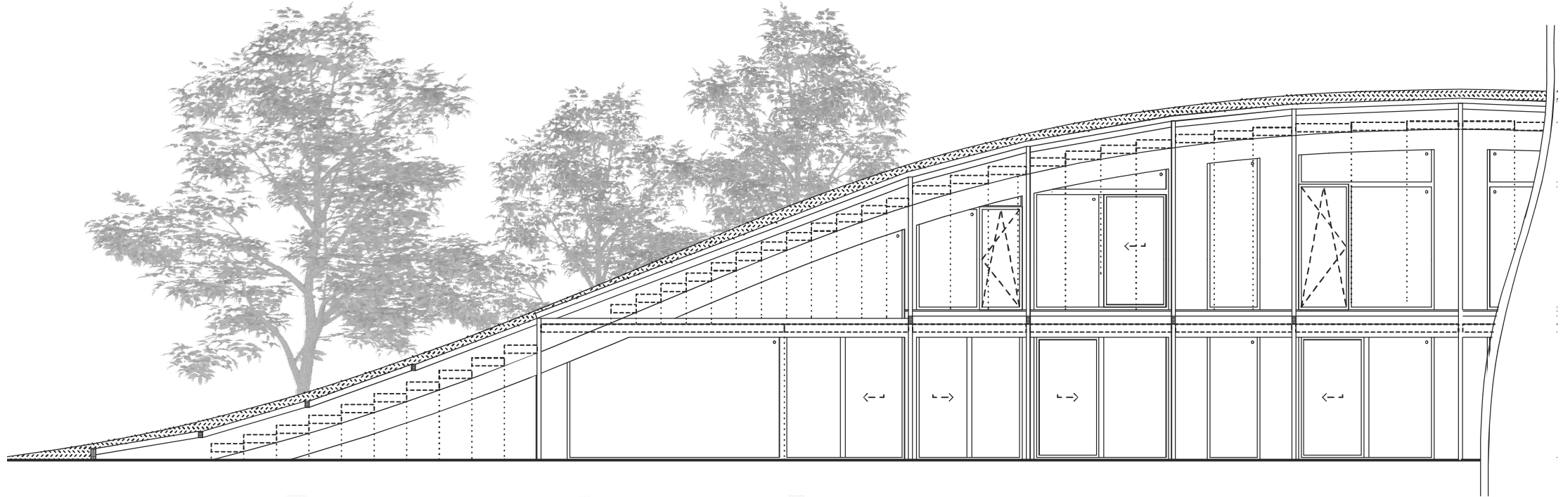
JIŽNÍ ŘEZO-POHLED - TECHNICKÝ
