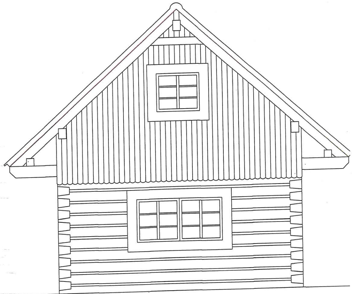
POHLED OD ZÁPADU
