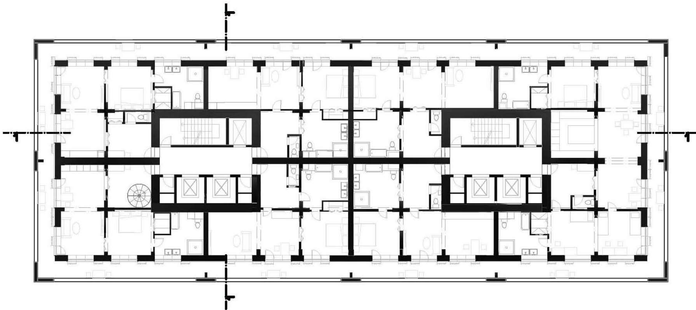
PŮDORYS TYPICKÉHO PATRA S PAVLAČÍ, M 1:200
