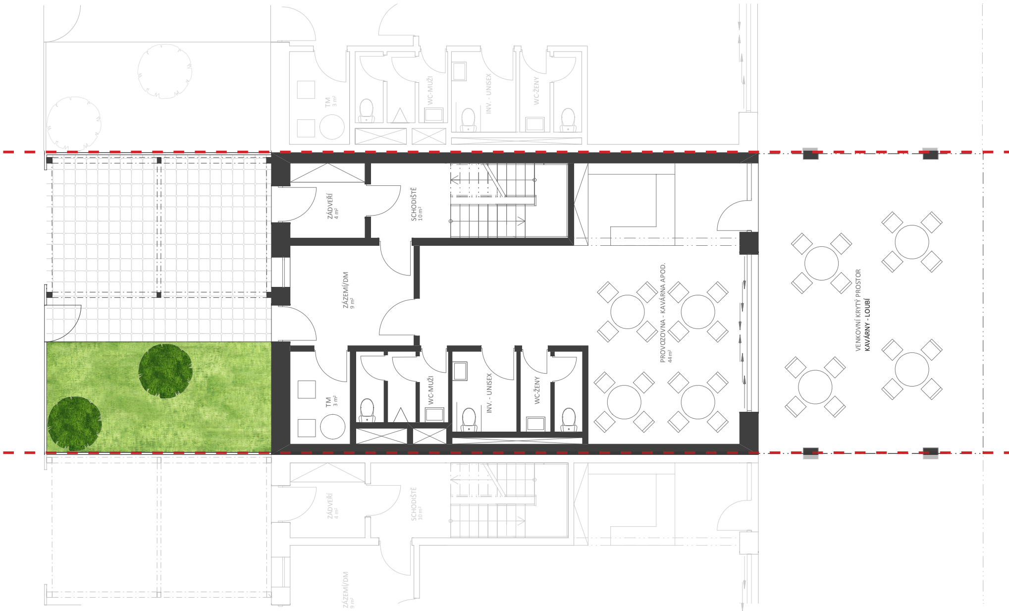
ŘADOVKA S-J - PŮDORYS 1.NP
