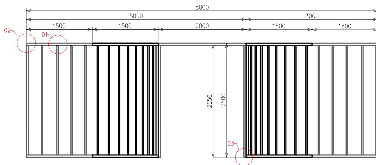
KONSTRUKCE B
