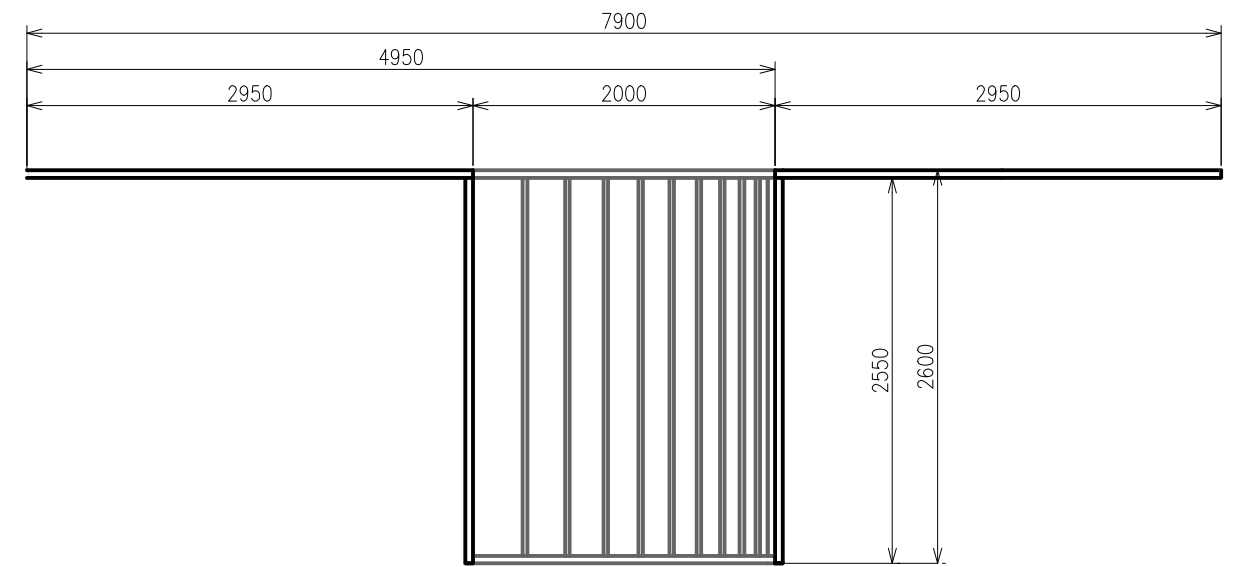
KONSTRUKCE C
