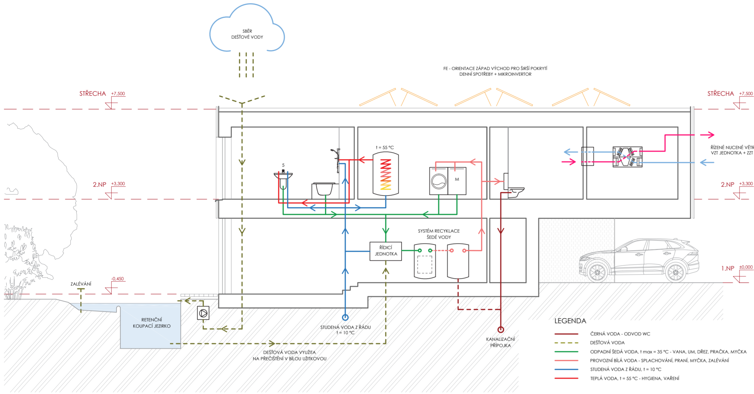
SCHÉMA VODNÍHO HOSPODÁŘSTVÍ
