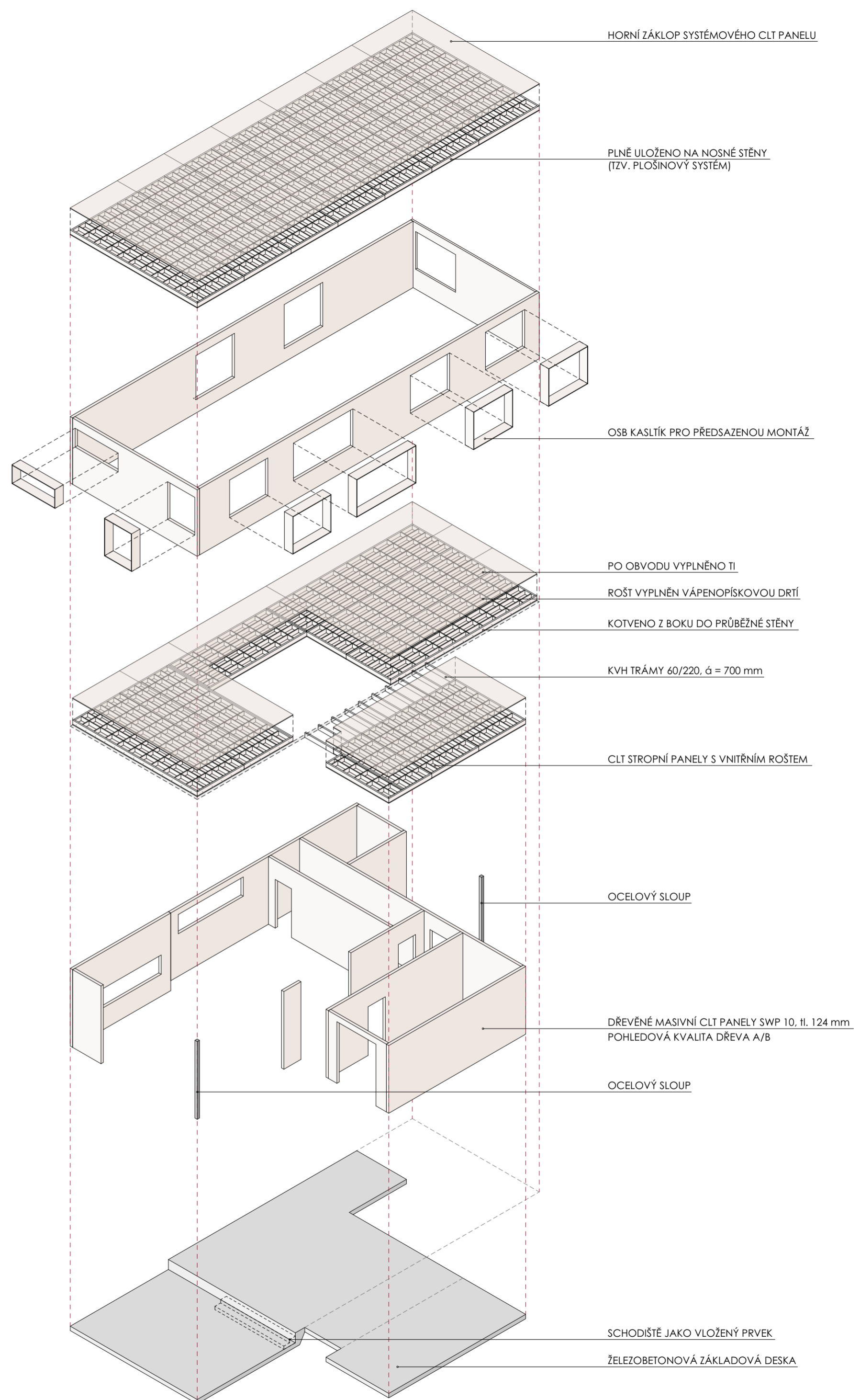
KONSTRUKČNÍ AXONOMETRIE
