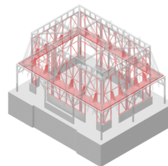
vnitřní rošť stěny a LVL konstrukce, která kompenzuje horizontální síly
