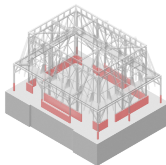
nový sokl pro přenos vertikálních sil
