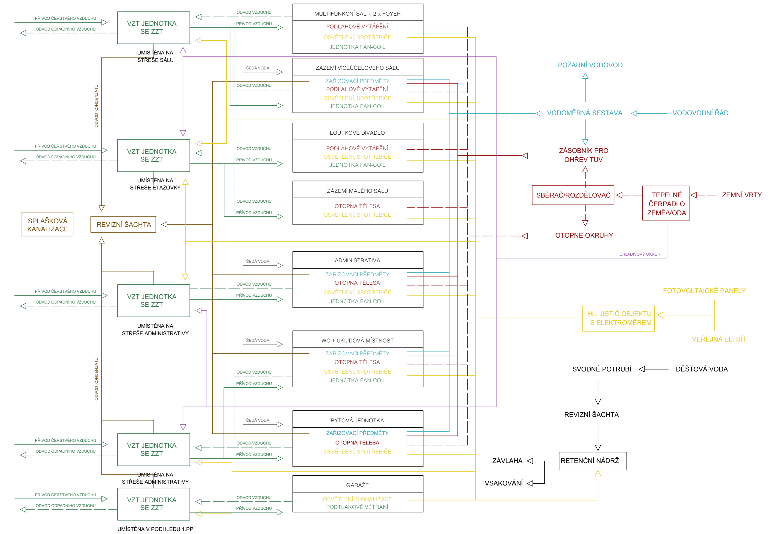
konceptní schéma I TZB část
