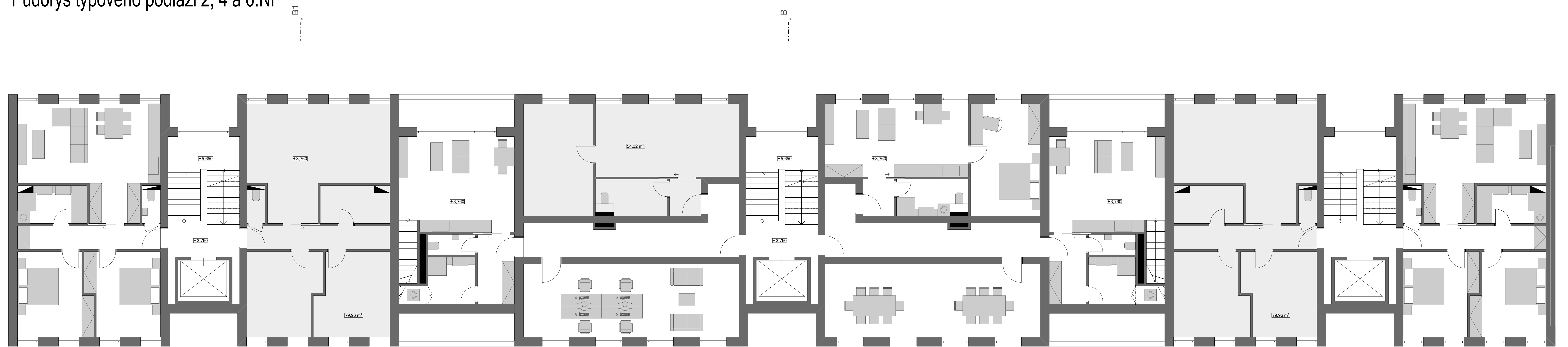
Půdorys typového podlaží 2, 4 a 6.NP
