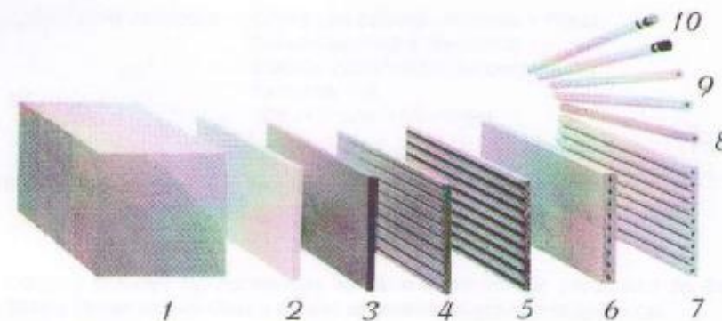
Schéma postupu výroby tužek ( http://crossasantagroup.com/pencil-resources.php )
